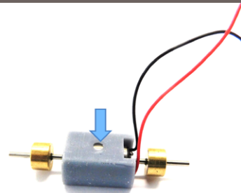
Der Motor wird mit Epoxidkleber oder Sekundenkleber in den Motorhalter eingeklebt The motor is glued into the motor holder with epoxy glue or super Glue
