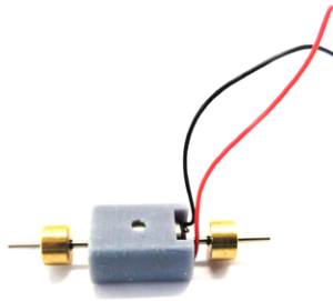
Platzieren der Motor in den Motorhalter Place the motor in the motor holder
